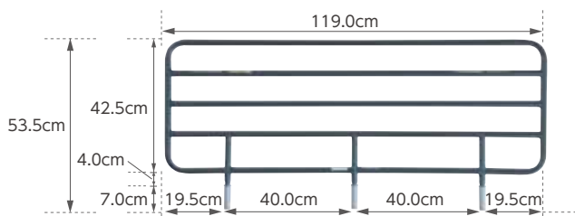
ロングサイドレール(1本入)
