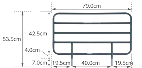
レギュラーサイドレール(2本組)
