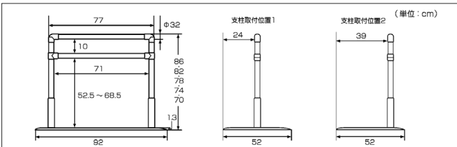
支柱取付位置:1(中央)
