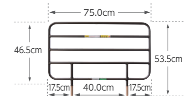
レギュラーサイドレール(2本組)
