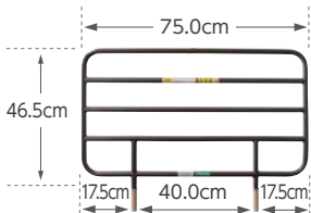
レギュラーサイドレール(2本組)
