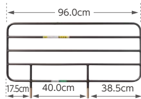
ロングサイドレール(2本組)
