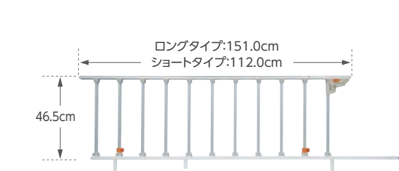
ロングタイプ (1本入)
