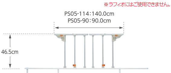
セパレートタイプ (1本入)
