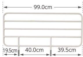
ロングサイドレール(2本組)
