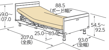
■ 固定脚 (83cm幅) (単位:cm)
