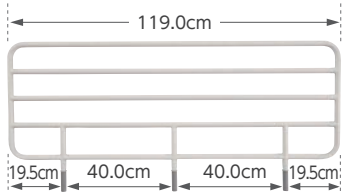
ロングサイドレール(1本)
