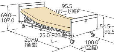
■ 4輪ロック [8cm径] (90cm幅) (単位:cm)
