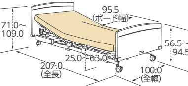
■ 4輪ロック [8cm径] (90cm幅) (単位:cm)
