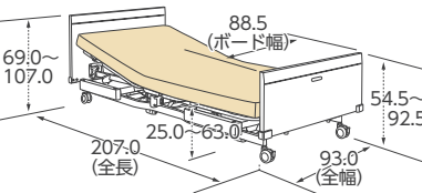
■ 4輪ロック [8cm径] (83cm幅) (単位:cm)
