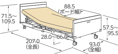
■ 4輪ロック [10cm径] (83cm幅) (単位:cm)
