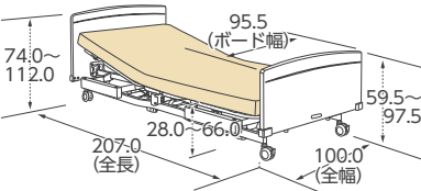
■ 4輪ロック [10cm径] (90cm幅) (単位:cm)
