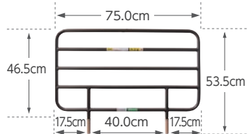
レギュラーサイドレール(2本組)
