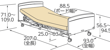
■ 4輪ロック [8cm径] (83cm幅) (単位:cm)
