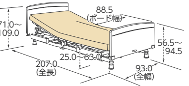
■ 固定脚 (83cm幅) (単位:cm)
