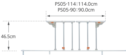
セパレートタイプ (1本)
